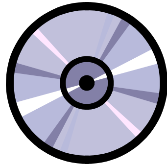
CD
