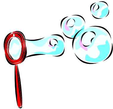
bubbles
