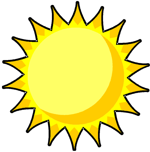
sun
